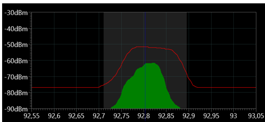
FM-радиостанция на частоте 92.8 MHz
